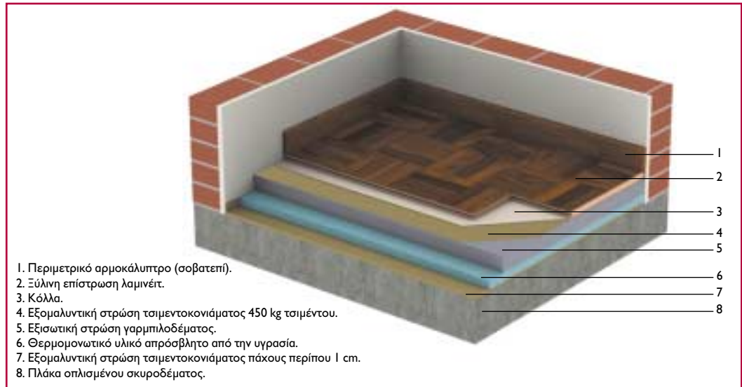
Κολλητό ξύλινο δάπεδο λαμινέιτ.
