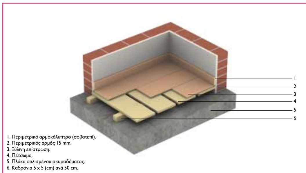
Καρφωτό ξύλινο δάπεδο με πέτσωμα.
