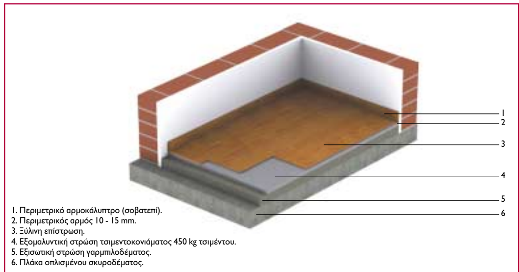
Επίστρωση επάνω σε πλάκα σκυροδέματος.
