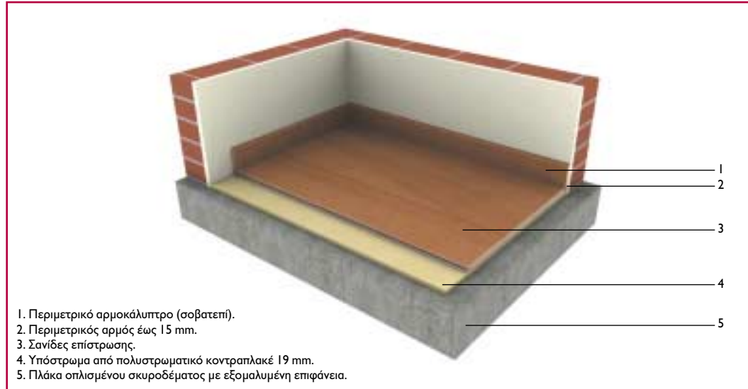
Καρφωτό ξύλινο δάπεδο επάνω σε πλάκες από πολυστρωματικό κοντραπλακέ.
