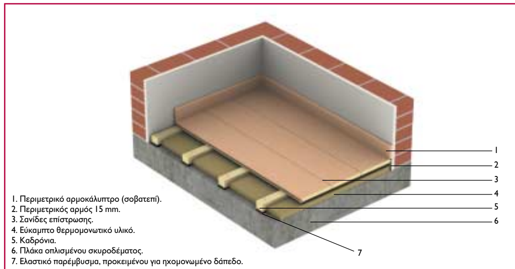
Καρφωτό ξύλινο δάπεδο επάνω σε καδρόνια.
