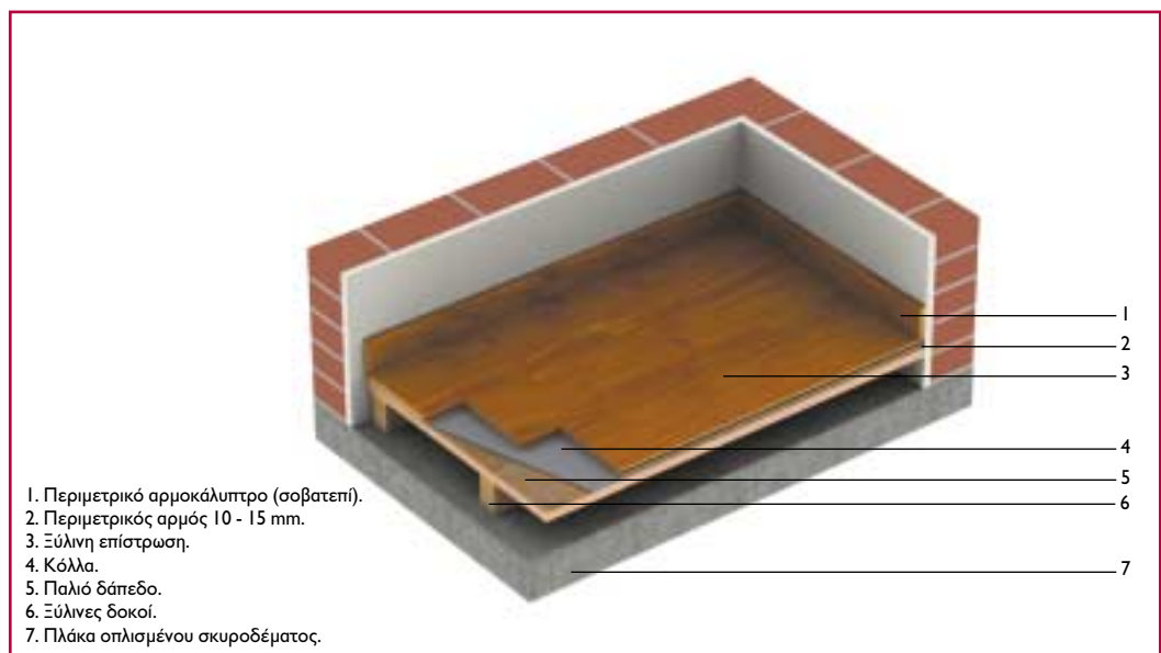
Επίστρωση επάνω σε παλιό καρφωτό ξύλινο δάπεδο.
