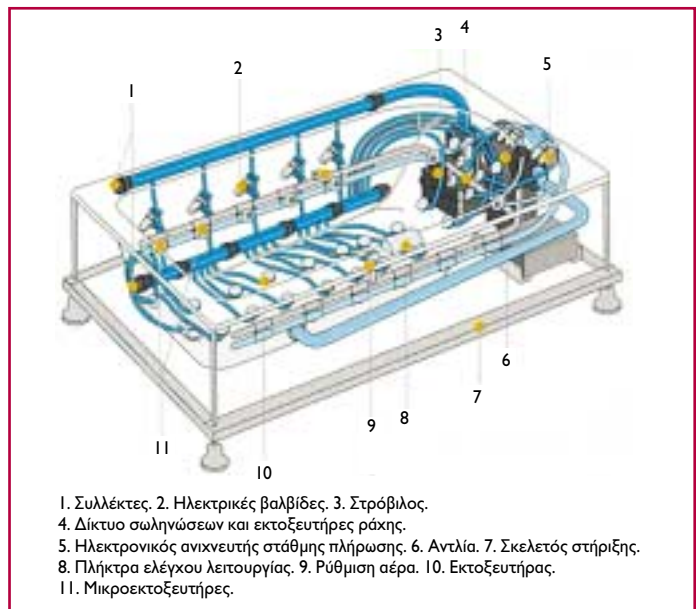
Μπανιέρα μεικτού συστήματος υδρομασάζ με εναλλασσόμενη ένταση.
