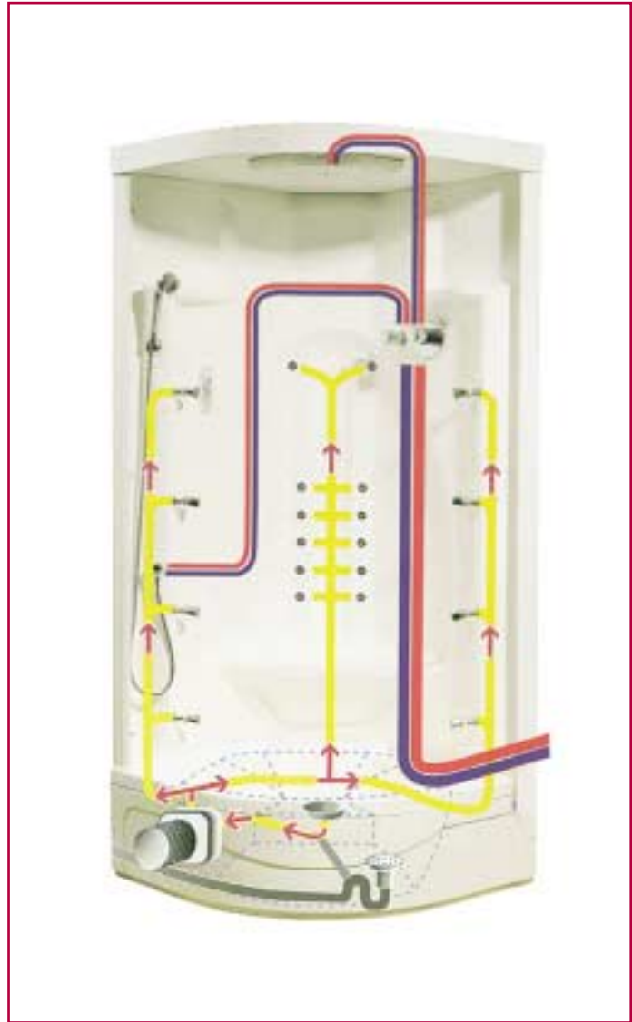
Δίκτυο σωληνώσεων σε καμπίνα ντους με σύστημα υδρομασάζ.
